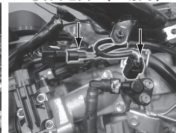
③インジェクター (2P カブラ)
