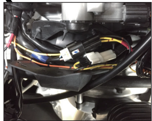
①クラクシャフトセンサー(ハーネスブーツ内) (ピックアップセンサー)(2Pカプラ)
