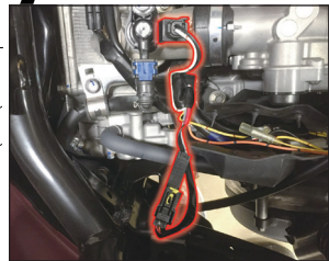
③インジェクター(2Pカプラ)
