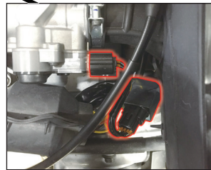
①クラクシャフトセンサー(ハーネスブーツ内) (ピックアップセンサー)(2Pカプラ)
