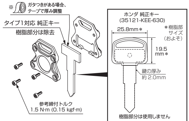
寸法図:タイプ1 ※表記はおおよその数値です。
