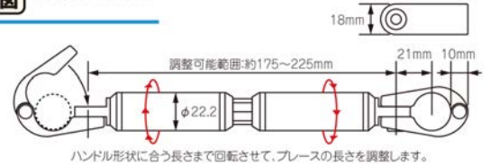
寸法図 HANDLE BRACE
