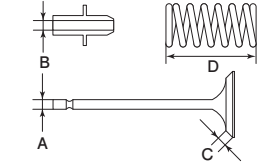
バルブ/バルブガイド/バルブスプリング
