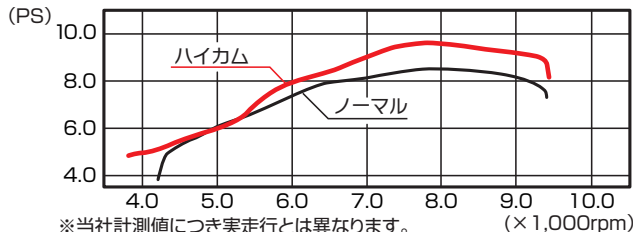
ハイカム装着時のパワー出力比較
